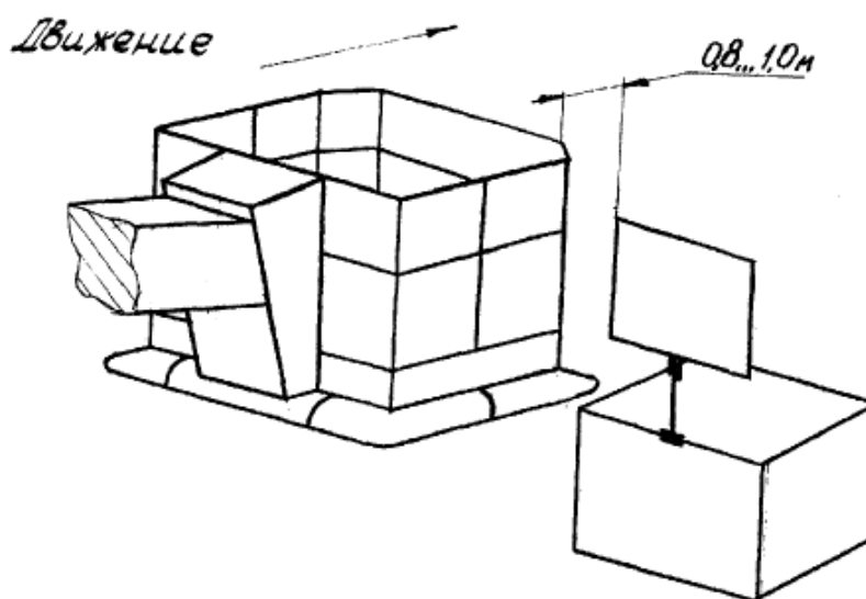
Рисунок 1. Схема положения люльки АПК относительно приспособления «цит-препятствие» при перемещении колен стрелы относительно друг друга
